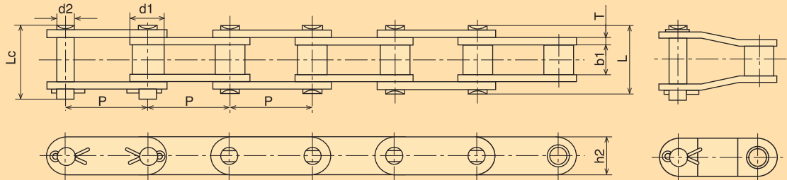
小滚子型 Small Roller Type
