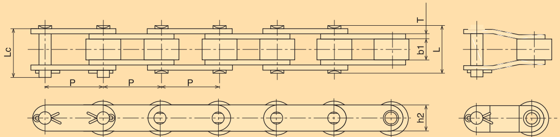
大滚子型 Large Roller Type
